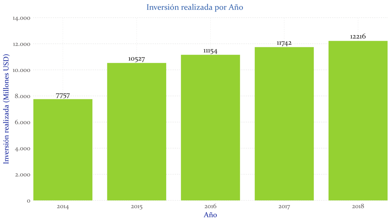
Gráfico 4: Inversión acumulada
